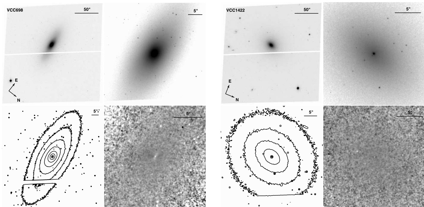
FIG. 25.— Left : VCC 698 (=NGC 4352, Hubble type S0_1(8) ). Right : VCC 1422 (=IC 3468, Hubble type E1,N: ). See Fig. 1 for details.
