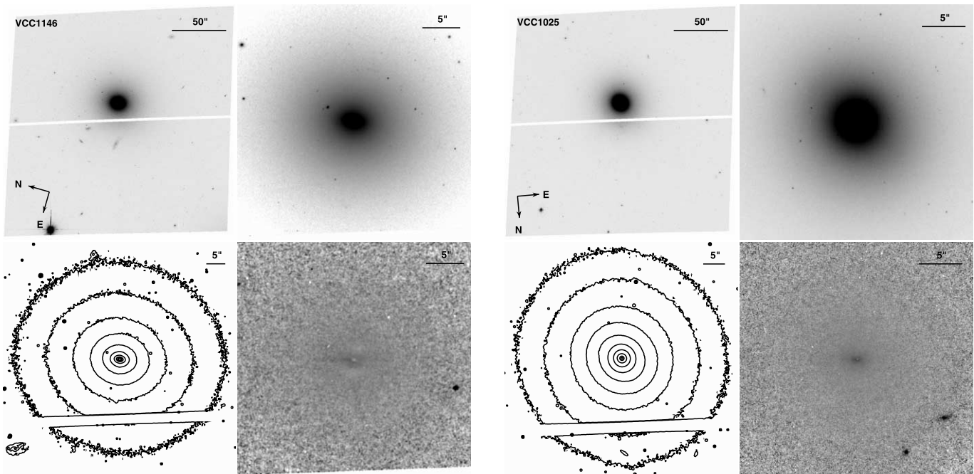
FIG. 20.— Left : VCC 1146 (=NGC 4458, Hubble type E1). Right : VCC 1025 (=NGC 4434, Hubble type E0/S0_1(0) ). See Fig. 1 for details.
