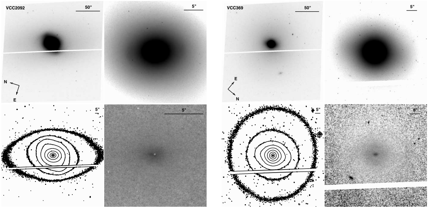
FIG. 8.— Left : VCC 2092 (=NGC 4754, Hubble type SB0_1(5) ). Right : VCC 369 (=NGC 4267, Hubble type SB0_1 ). See Fig. 1 for details.
