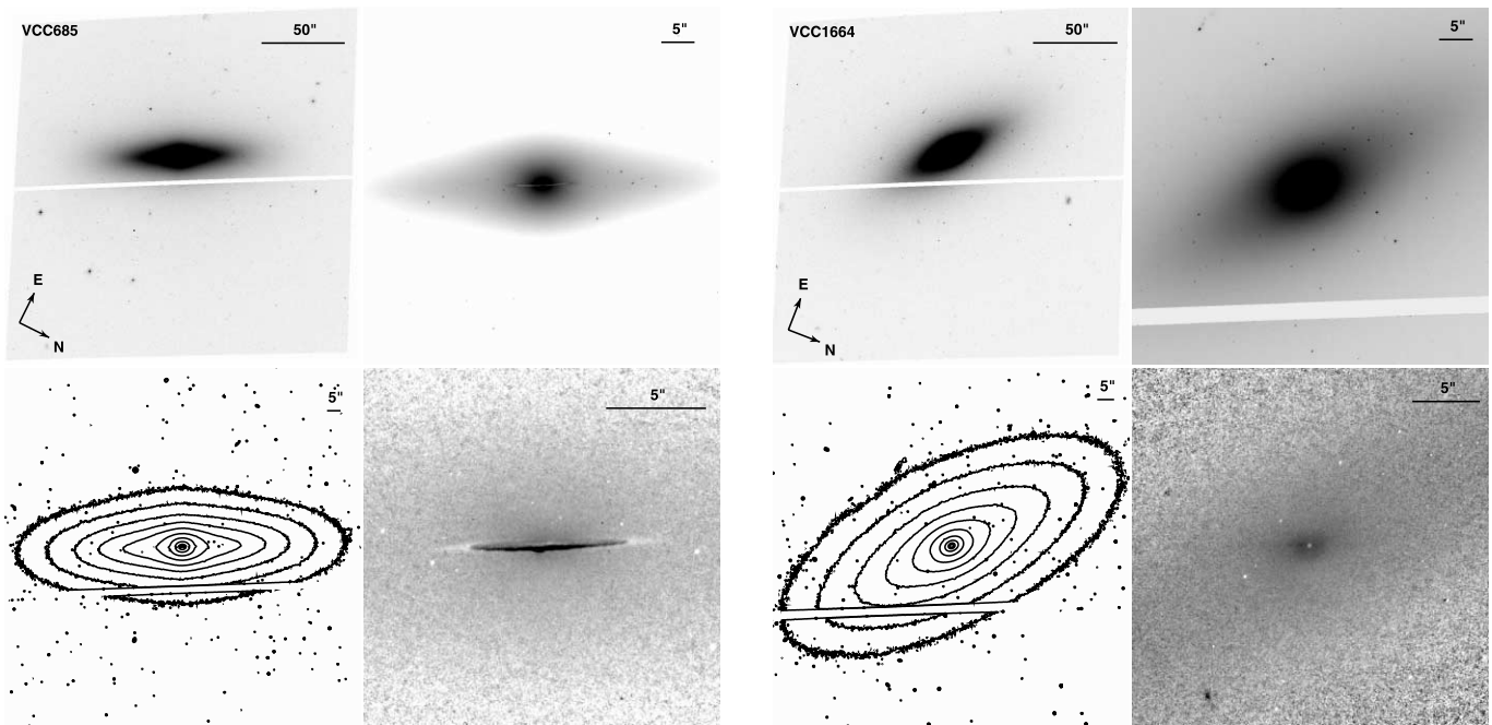
FIG. 11.— Left : VCC 685 (=NGC 4350, Hubble type S0_1(8) ). Right : VCC 1664 (=NGC 4564, Hubble type E6). See Fig. 1 for details.
