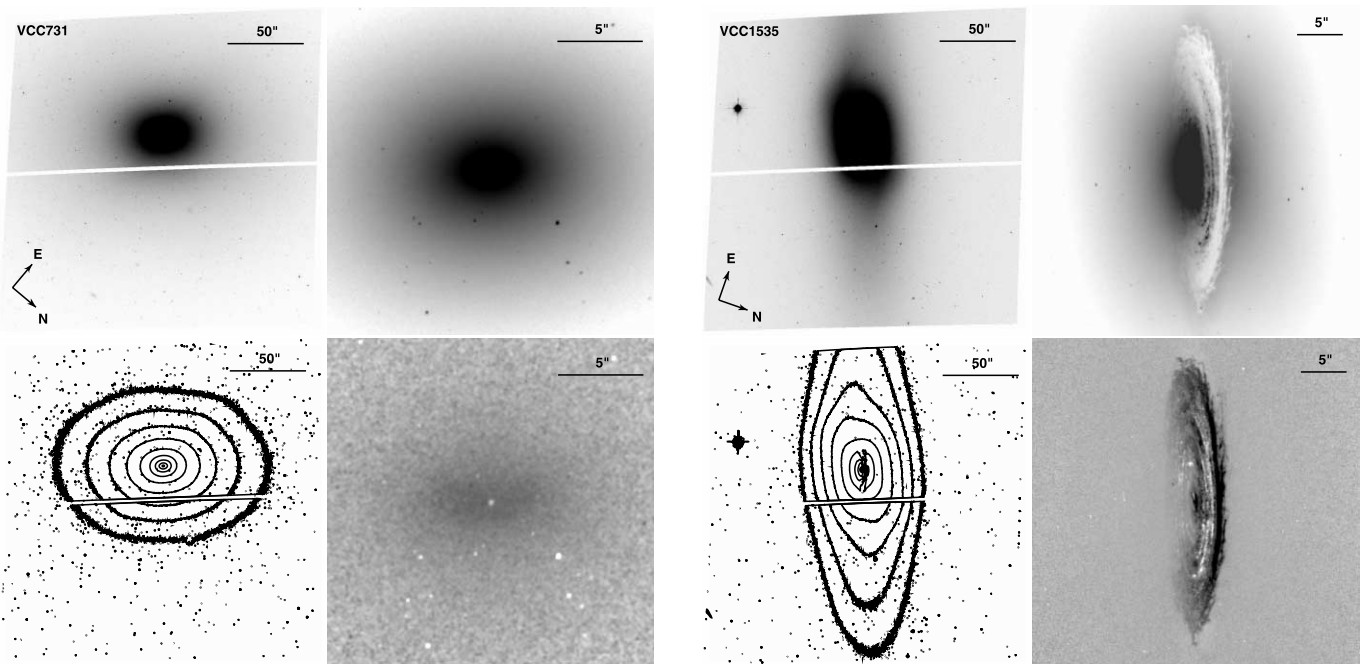
FIG. 4.— Left : VCC 731 (=NGC 4365, Hubble type E3). Right : VCC 1535 (=NGC 4526, Hubble type S0_3(6) ). See Fig. 1 for details.
