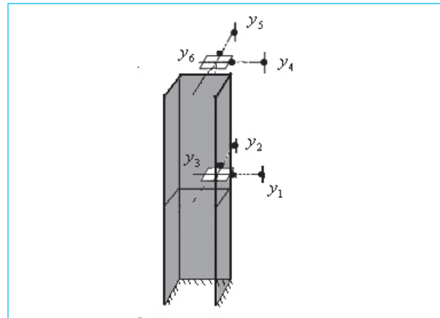
Figura 1.4 Subsistemas bases por rigidizador espacial
