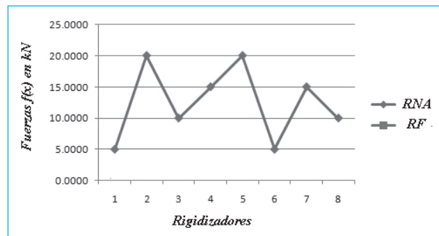
Gráfico 7 Fuerzas por rigidizadores en kN según los procedimientos considerados.
