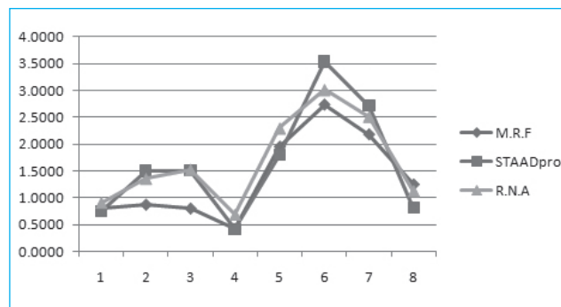
Gráfico 11 Desplazamientos por rigidizadores según los procedimientos considerados.
