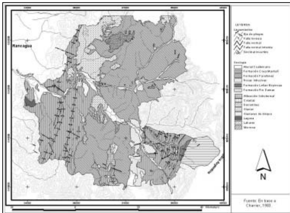
FIGURA N° 2 AMBIENTE MORFOTECTÓNICO Y ESTRUCTURAL, CORREDOR LAS LEÑAS
