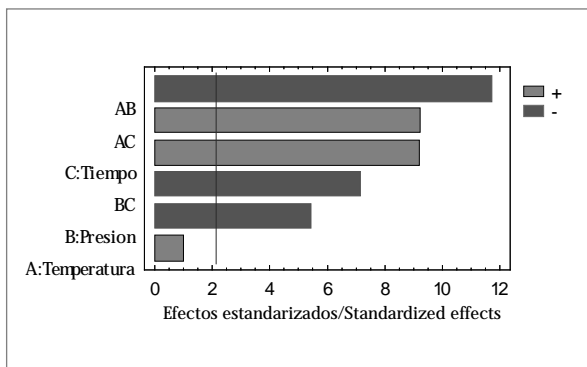
Figura 11. Análisis de Pareto para el espesor de las muestras Figure 11. Pareto analysis for sample thickness
