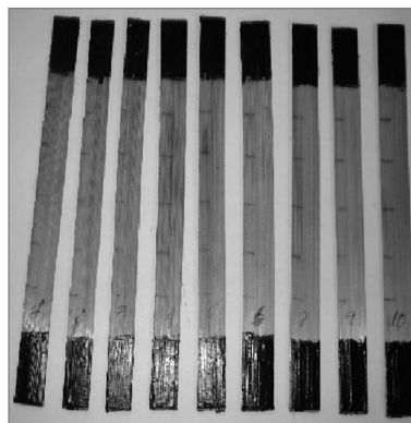
Figura 1. Probetas para ensayos de tracción Figure 1. Specimens for tensile tests
